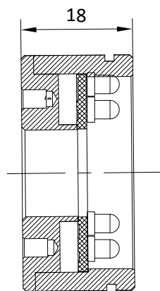
剖视图 B-B
