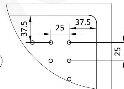
局部放大视图 I
